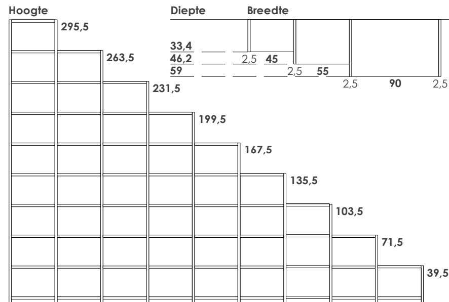
Studio-/Jeugdkamerinrichting
